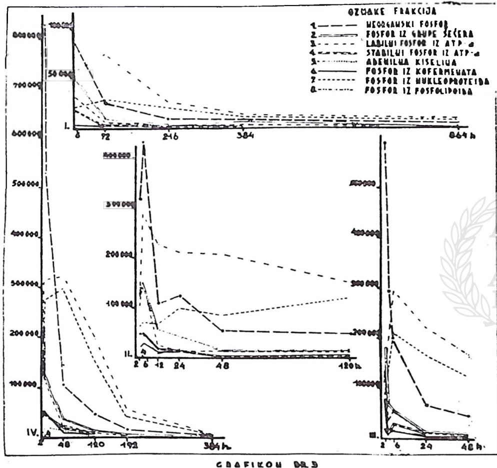
GRAFIČKI PRIKAZ KRETANJA RADIOFOSFORA U ORGANSKIM FOSFOROVIM JEDINJENJIMA U JETRI PACOVA
